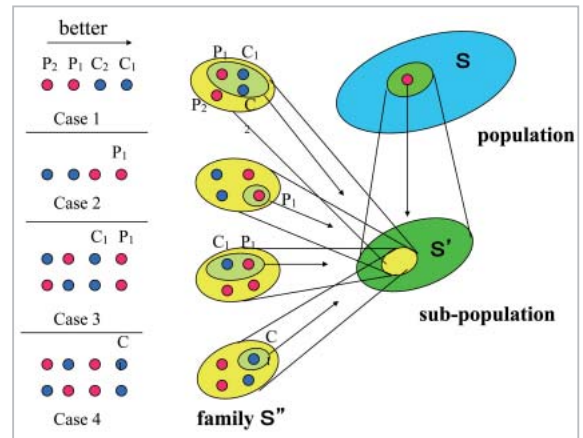
図18 PfGA における集団と選択ルール
