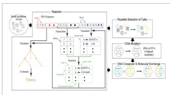
図40 CGP アルゴリズム
