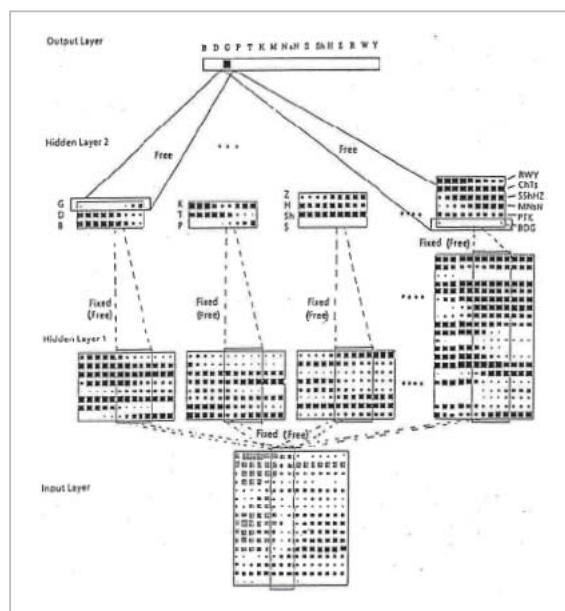
図10 全子音ネットワークのモジュール構成
