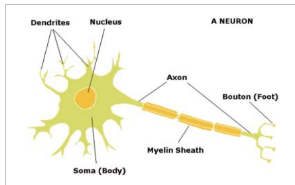
図3 ニューロン（神経細胞）
