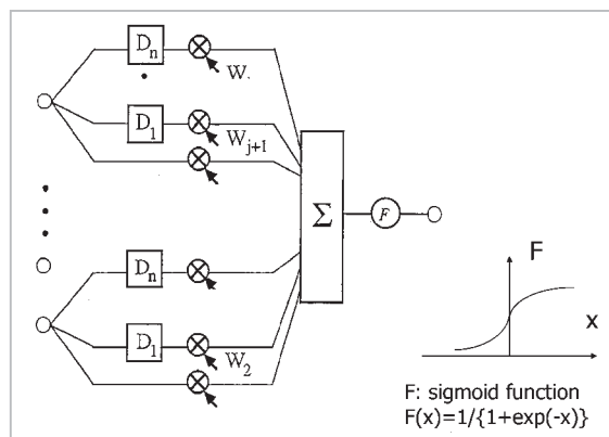
図8 時間遅れ神経回路網 (TDNN) のユニット
