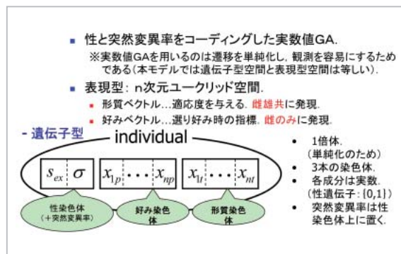
図26 性選択の提案モデル
