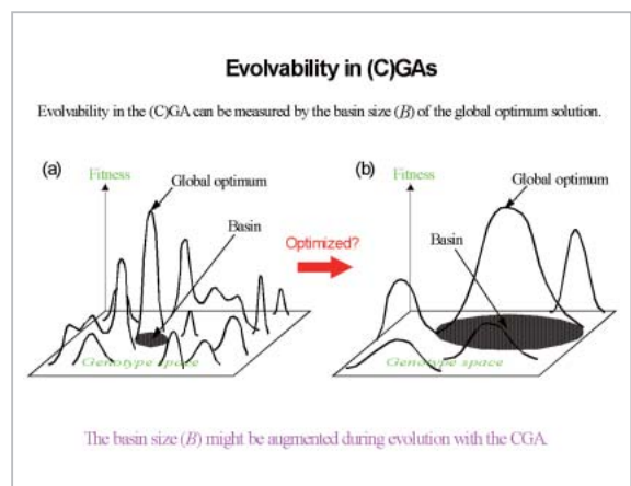
図32 C (GA) における進化可能性
