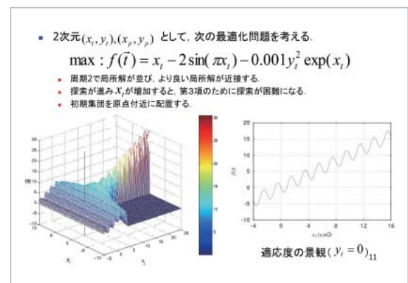
図27 例題による提案モデルの検証
