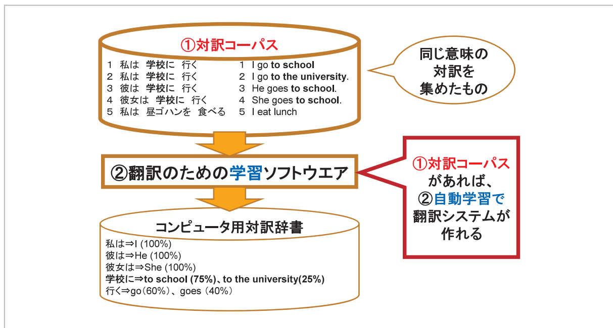
図 2 コーパスベース翻訳技術の基本
