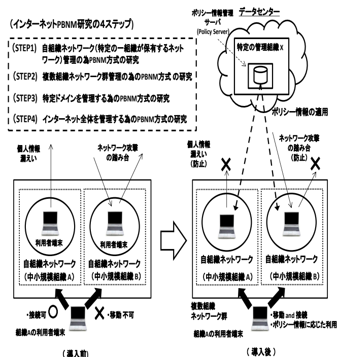
図1 インターネットPBNM
