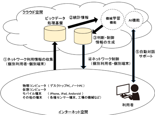
図4 AI・機械学習を活用する特定ドメインの新規管理手法
