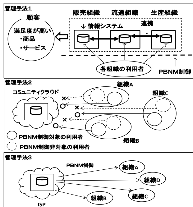
図6 PBNM管理手法
